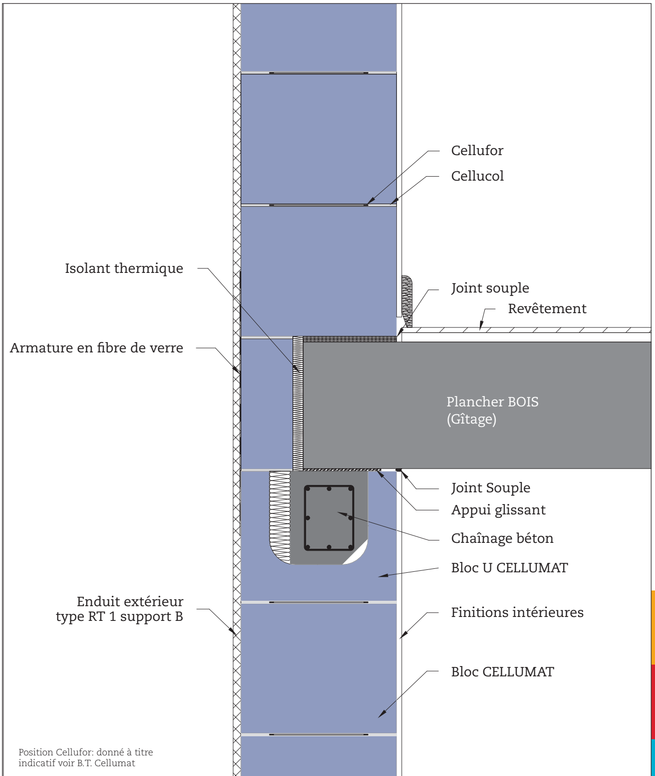
Détail: mur massif - appui gîtage
