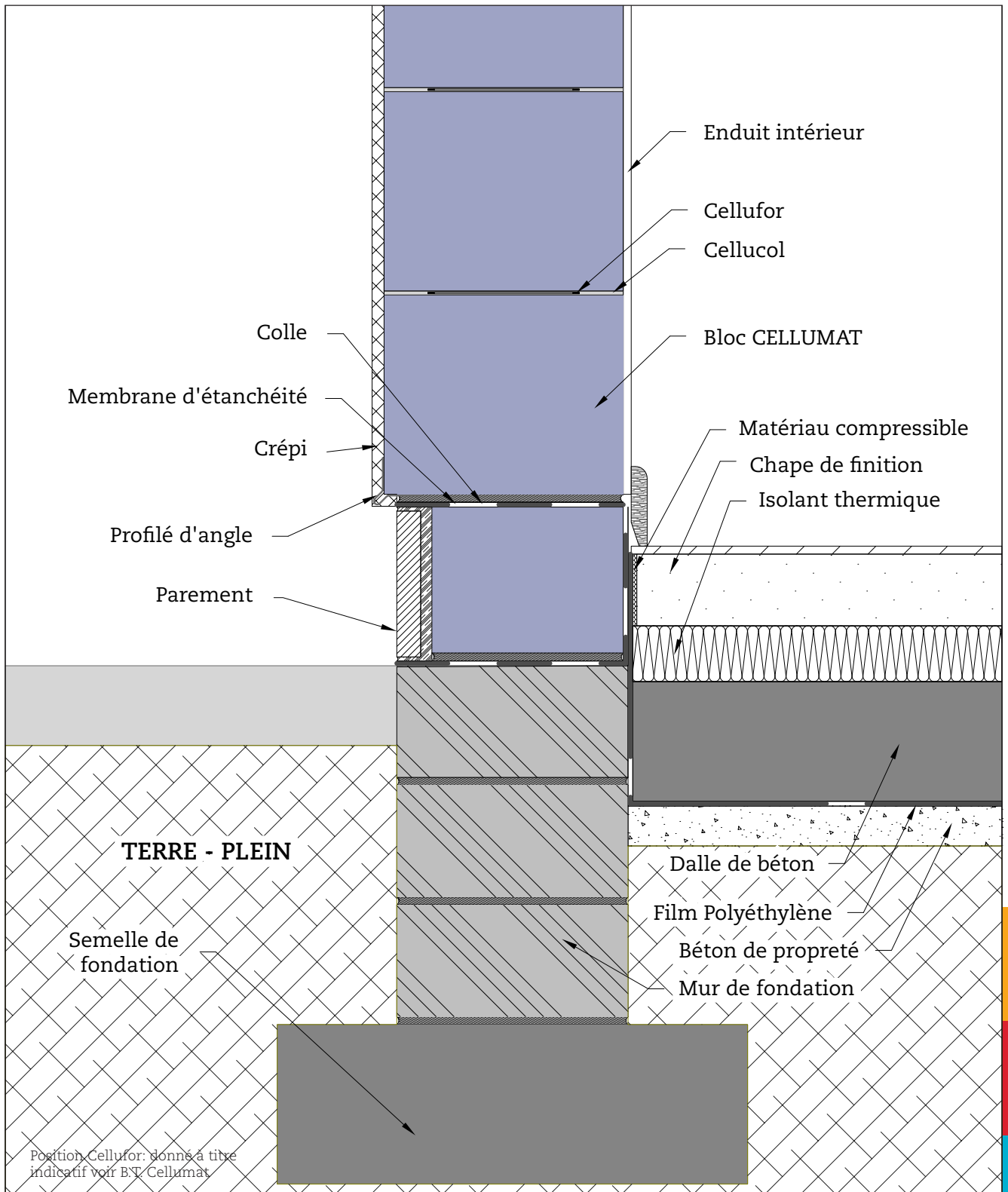
Detail: mur massif - détail en pied - pose sur fondation
