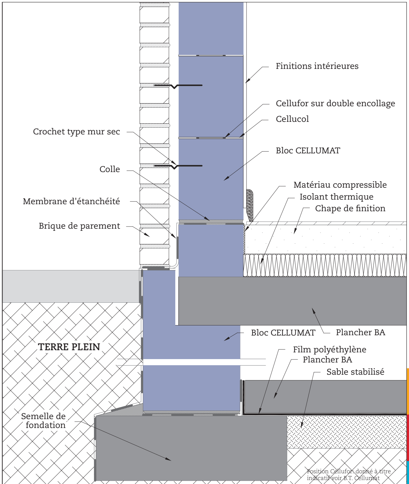
Détail: mur double - détail en pied - pose sur plancher béton
