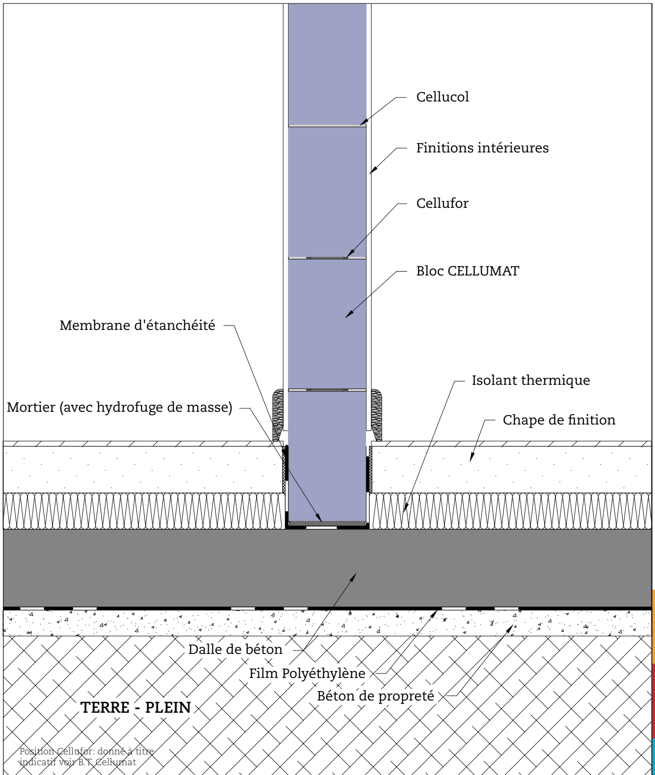
Détail: mur intérieur - porteur sur dalle béton
