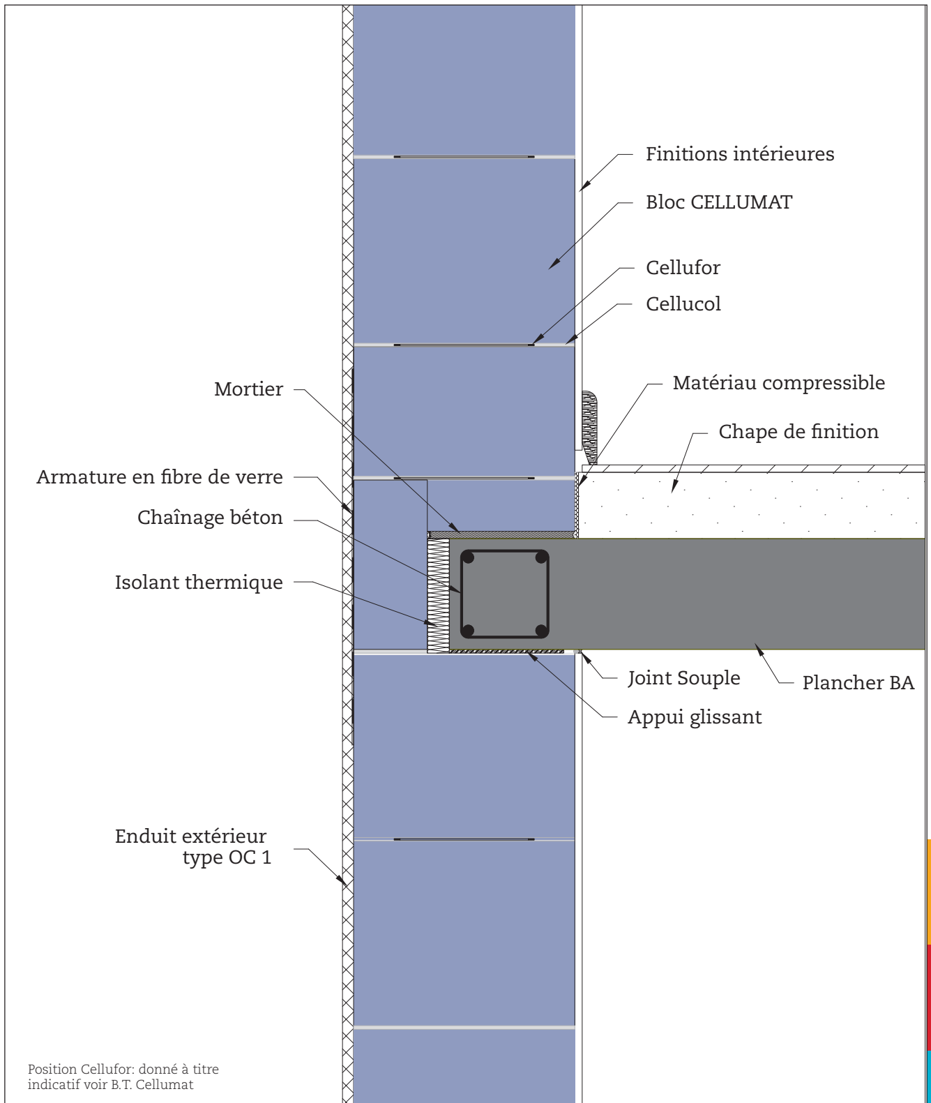
Détail: mur massif - appui plancher étage
