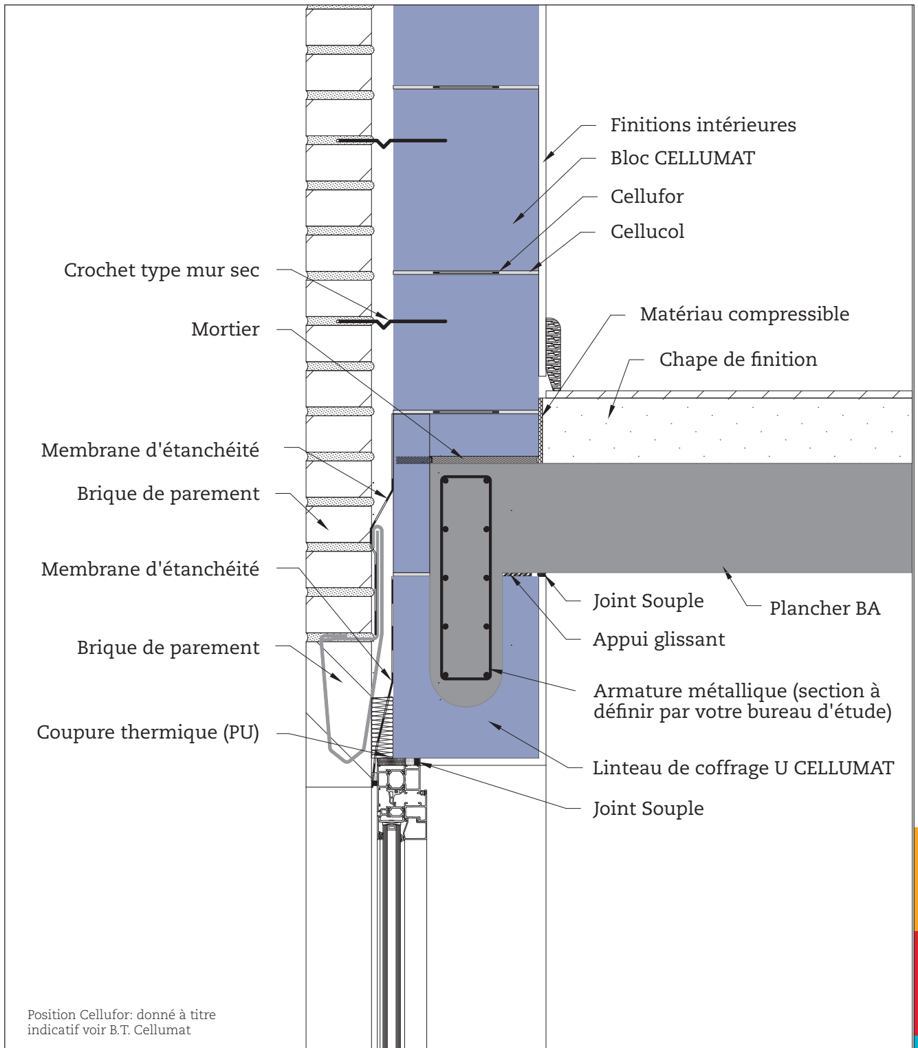
Détail: mur double - linteau de coffrage U liaison dalle - linteau avec armature métallique
