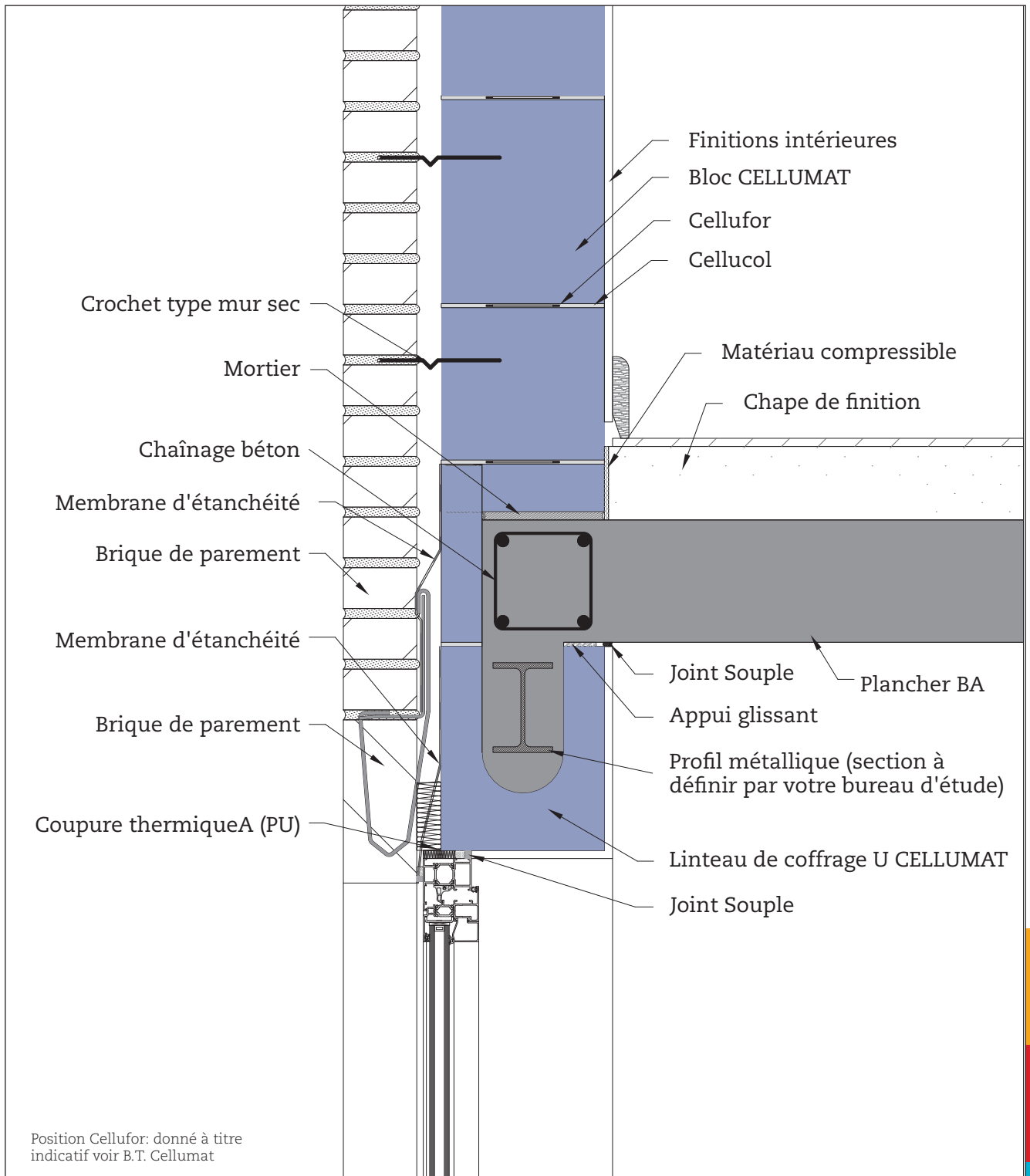
Détail: mur double - linéau de coffrage U liaison dalle - linéau avec profil métallique
