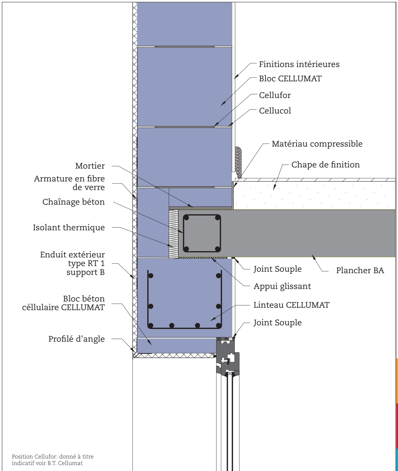
Détail: mur massif - appui plancher béton sur linteau Cellumat
